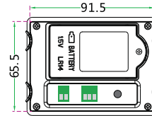
底视图 Bottom view
